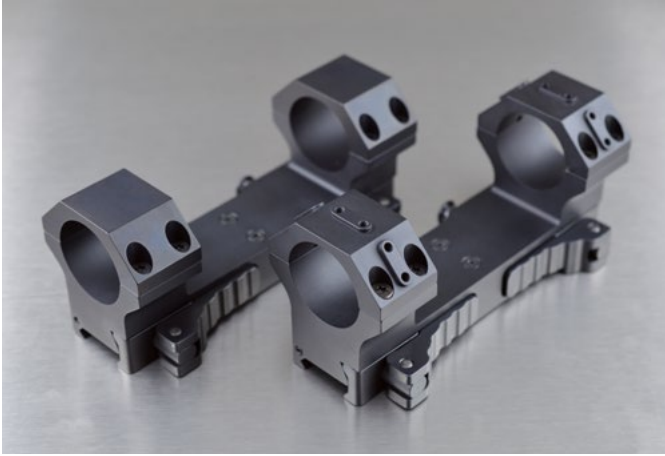
Abbildung zeigt Schnellspannmontage mit und ohne Universalschnittstelle Picture shows quick release mounting with and without universal interface
